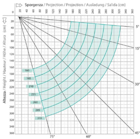
Diagramma di copertura a parete
