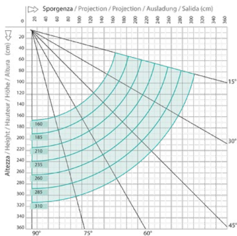
Diagramma di copertura a soffitto
