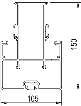
Viga estándar para puerta de vidrio
